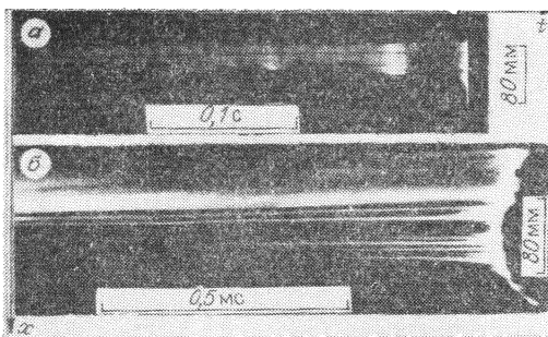
Рис. 1. Фоторегистрограммы взрывного процесса при поджигании от открытого торца.
