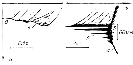
Рис. 2. Общая схема взрывного процесса при поджигании от открытого торца.
